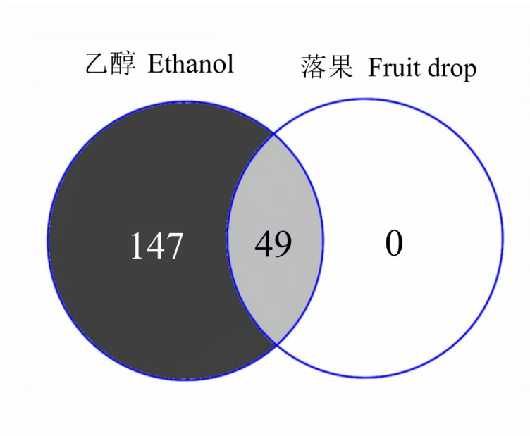
附图 1 WGCNA 模块基因数量 S1 The number of WGCNA module genes
